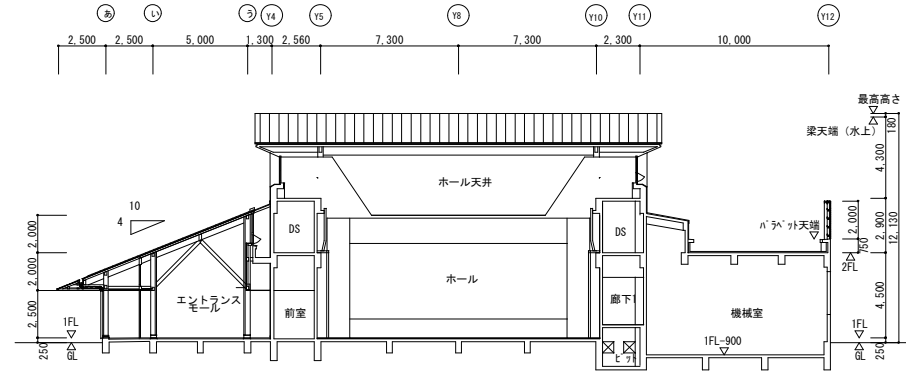
C断面図
