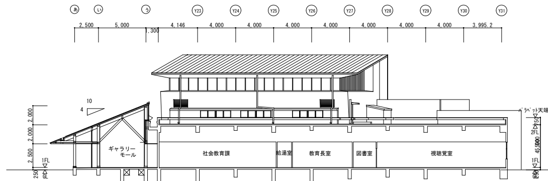
I断面図
