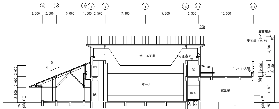
E断面図
