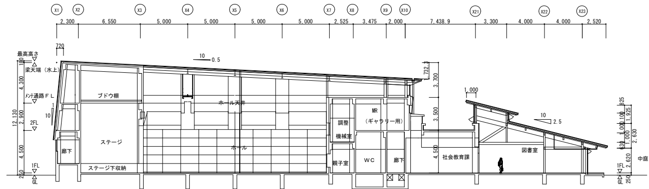
A断面図
